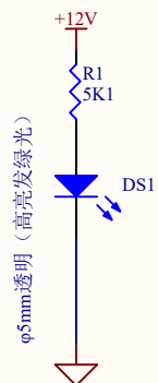
电源
