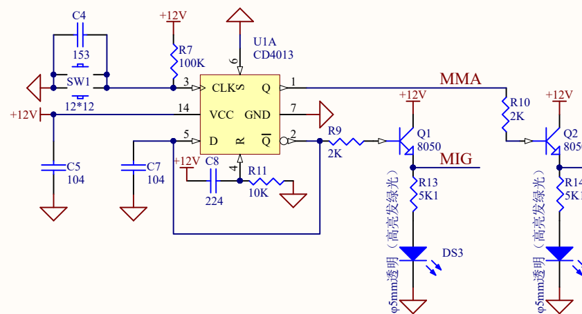
MMA/MIG转换
