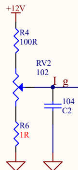
电流给定
