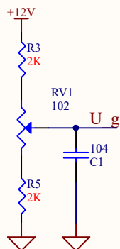
电压给定
