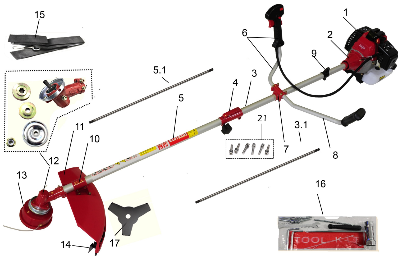
Схема: Штанга и привод
