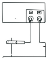
Схема сварки с прямой полярностью
