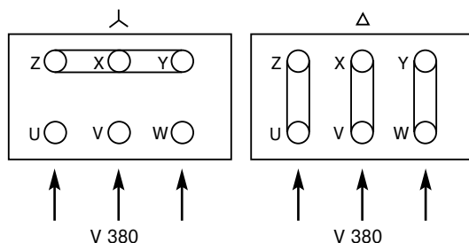
рис. 2 Подключение к электросети
